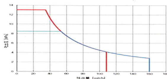
ポンプ能力線図
