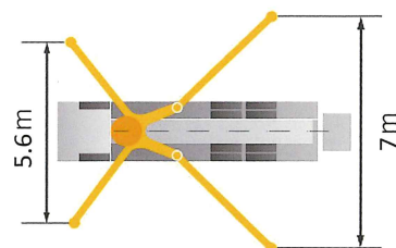
アウトリガー展開図+ワンサイドサポート(OSS)
